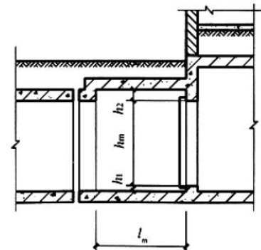
b) 剖面图
