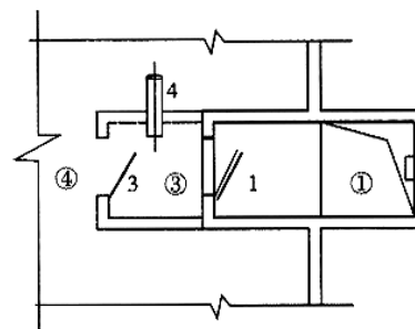
b) 主体允许染毒的通风口
