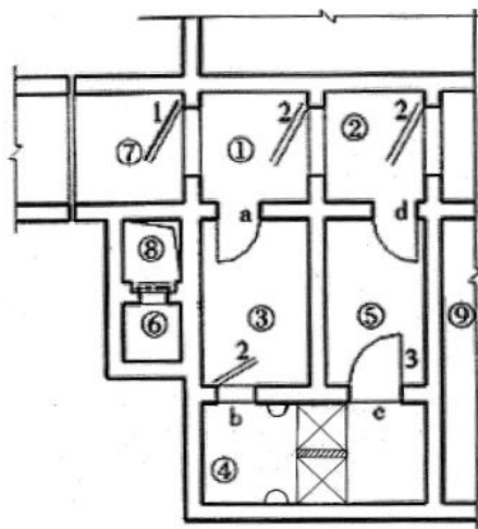
图 3.3.23 洗消间平面
