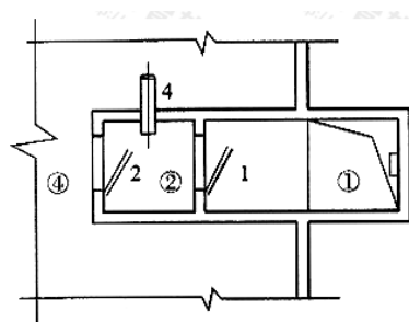
a) 主体要求防毒的通风口
