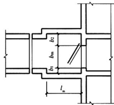
a) 平面图
